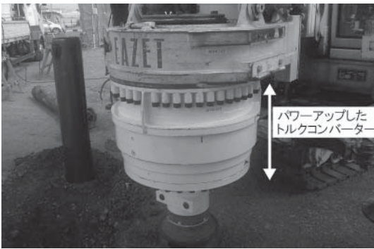
■トルクコンバーター部分
